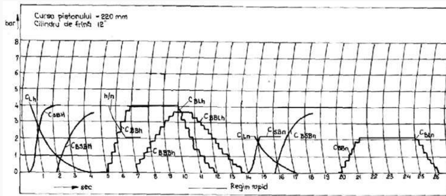
CURBELE DE PRESIUNE ETALON PENTRU DU 15 3,6-2,1/4 BAR (LE 5100 kW)
